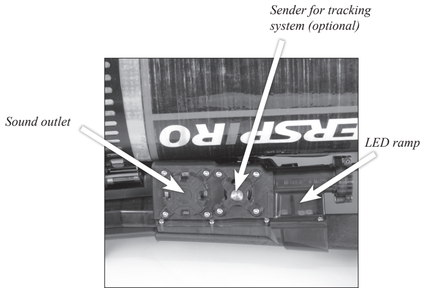
BAC unit, left side shown
